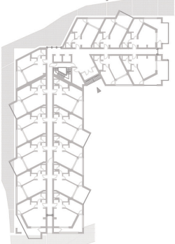
Osnova 2. Sprata
