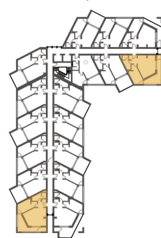
Osnova 3. Sprata
