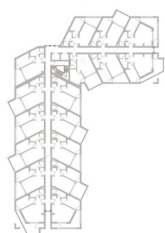
Osnova 4. Sprata
