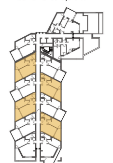
Osnova 5. Sprata
