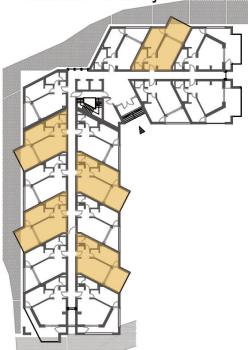
Osnova 2. Sprata
