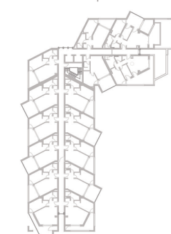
Osnova 4. Sprata
