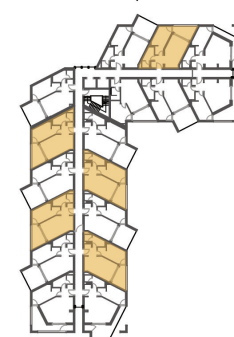
Osnova 3. Sprata
