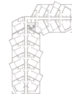
Osnova 4. Sprata
