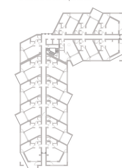
Osnova 2. Sprata
