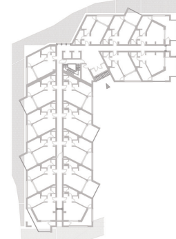
Osnova 2. Sprata
